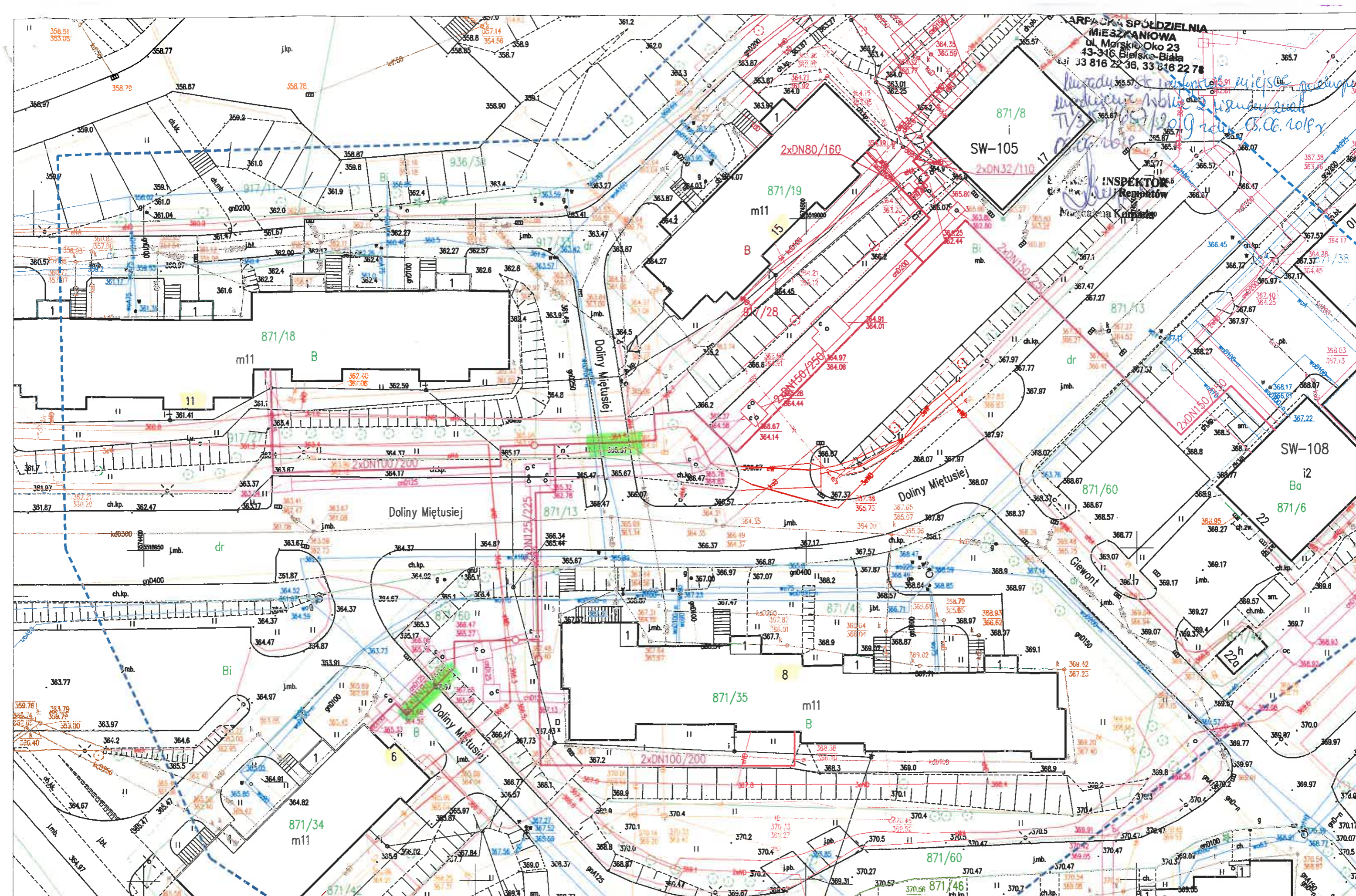
Budowa osiedlowej sieci ciepłowniczej w technologii rur preizolowanych 2 x DN150/250 - 32/110mm od SW-108 przy ul.Giewont 22 do budynków mieszkalnych wielorodzinnych przy ul.Giewont 6, ul.Doliny Miękusiej 8,11,15 oraz obiektu SW-105 przy ul. Doliny Miękusiej 17 w Bielsku-Białej.
